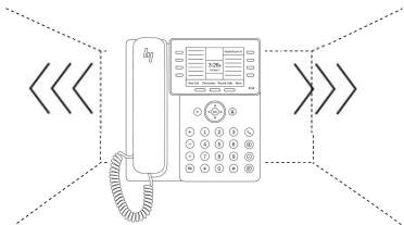
NoiseBlockAI v3
